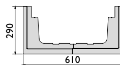
Káblový žľab KK 3, s vloženým krytom, L = 1000 mm
