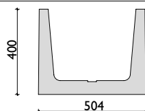
Káblový žľab WL, s položeným krytom L = 1000 mm
