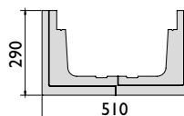
Káblový žľab KK 2, s vloženým krytom, L = 1000 mm
