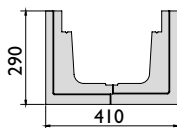
Káblový žľab KK 1, s vloženým krytom, L = 1000 mm
