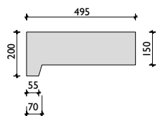
Deliaca stienka, L = 495 mm
